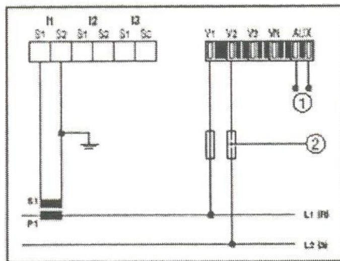
Двухфазная сеть (2BL)
