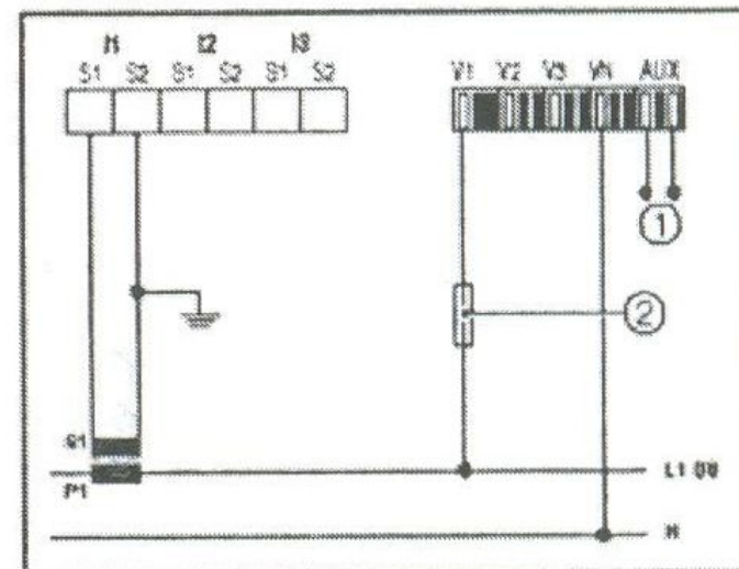
Однофазная сеть (1BL)
