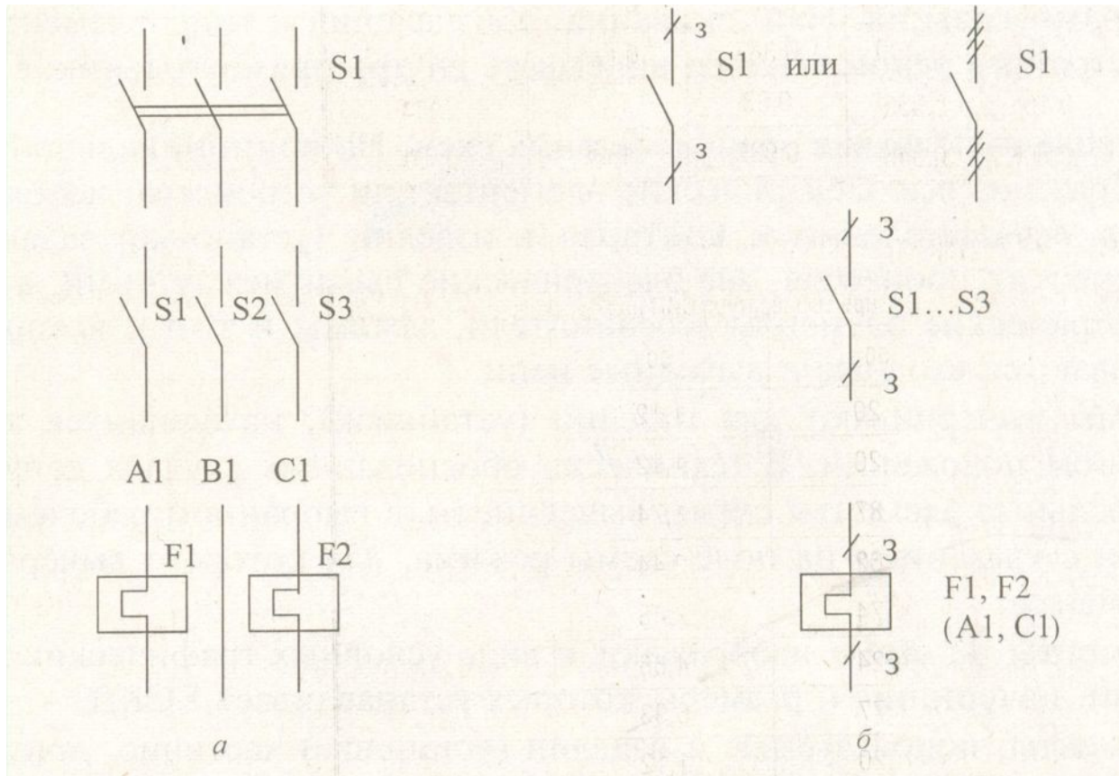
Примеры выполнения некоторых элементов в многолинейных (а) и однолинейных (б) схемах
