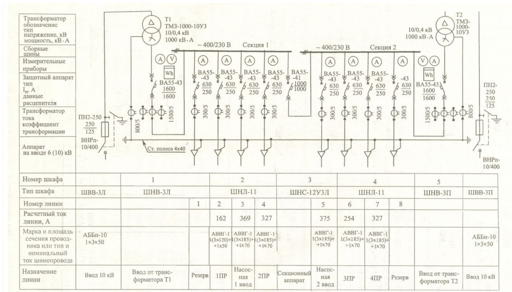
Пример выполнения принципиальной схемы КТП в соответствии с ГОСТ 21.613-88
