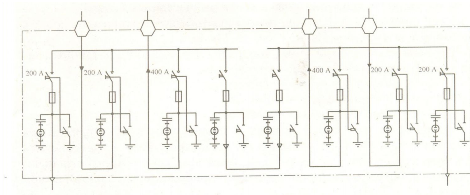
Принципиальная схема РУ10(6) кВ подстанции
