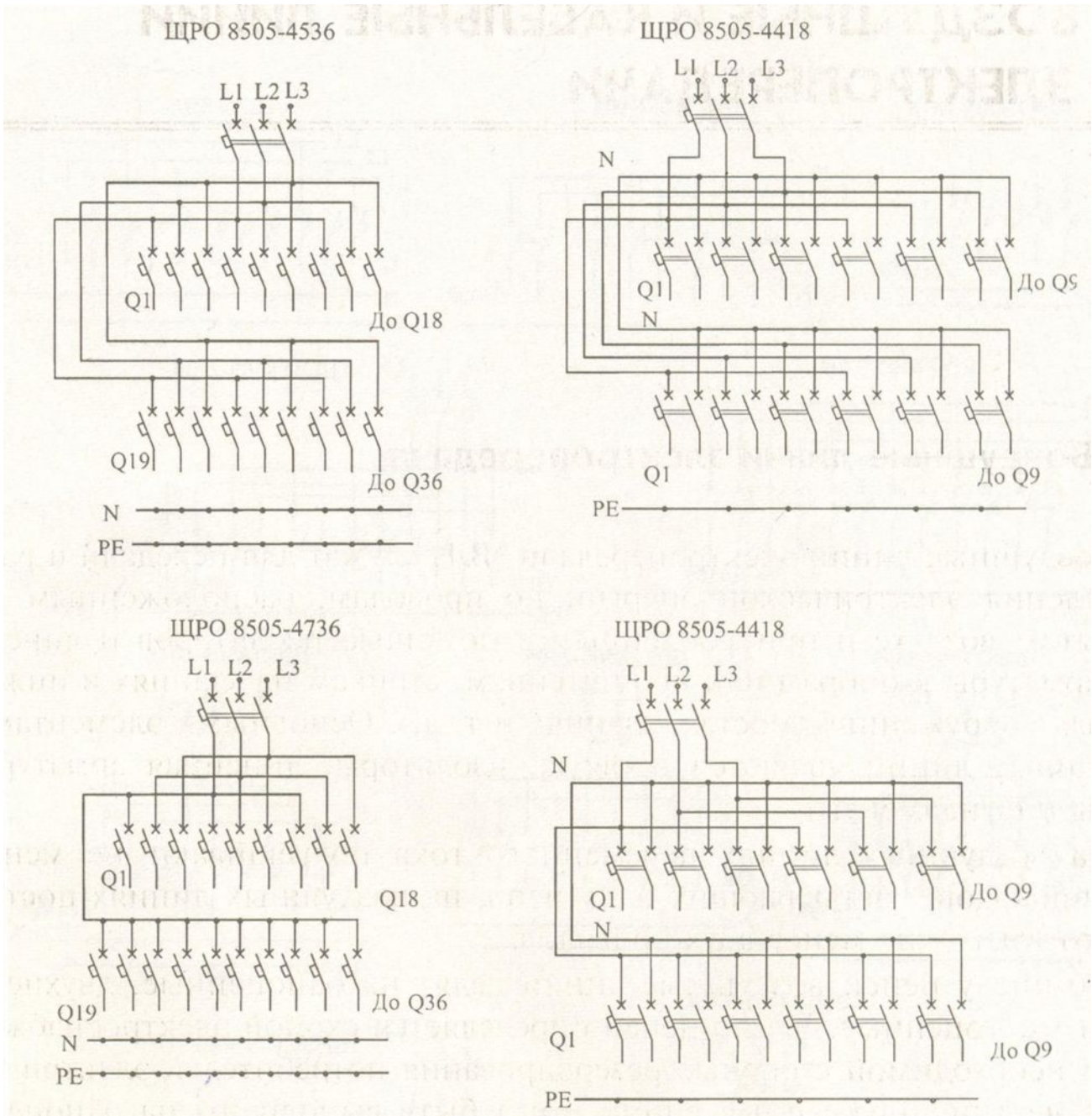
Принципиальные схемы ящика ЩРО8505 (часть 2)
