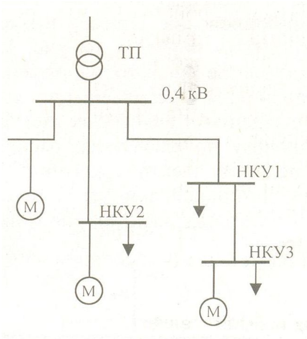
Радиальная схема распределения электроэнергии
