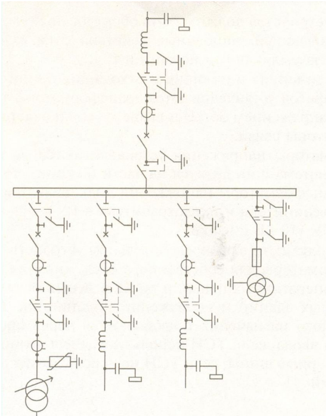
Схема с одной системой шин
