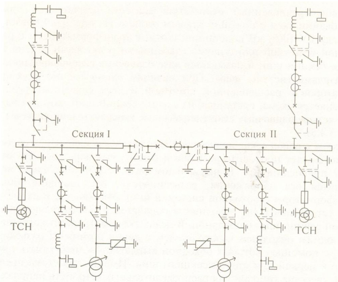
Схема с одной секционированной системой шин
