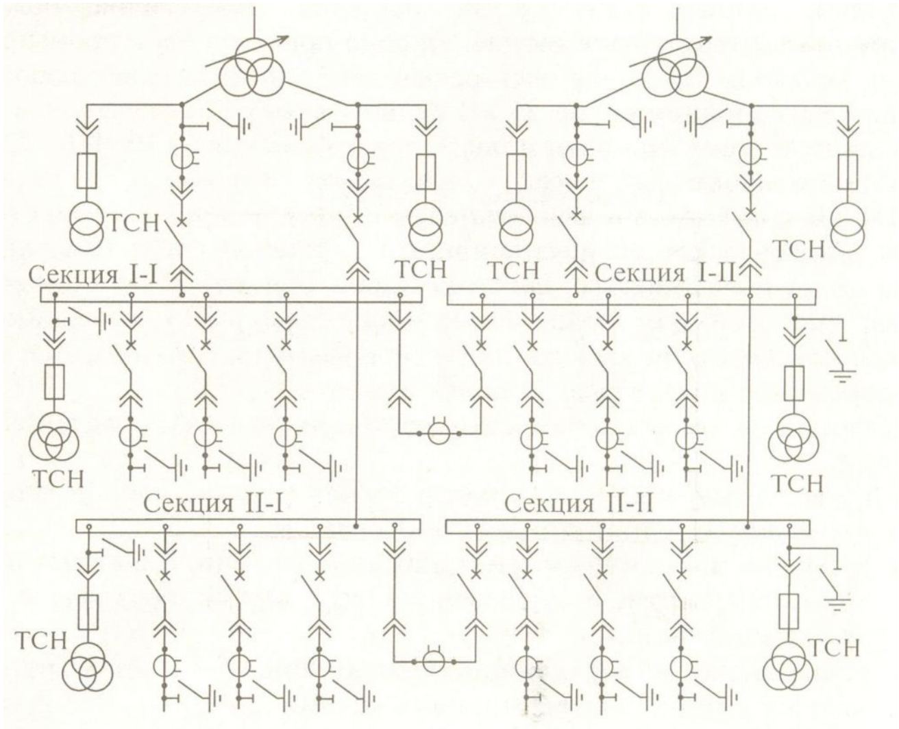
Схема с двумя одиночными секционированными системами шин (ТЧН при постоянном оперативном токе подключаются к сборным шинам)
