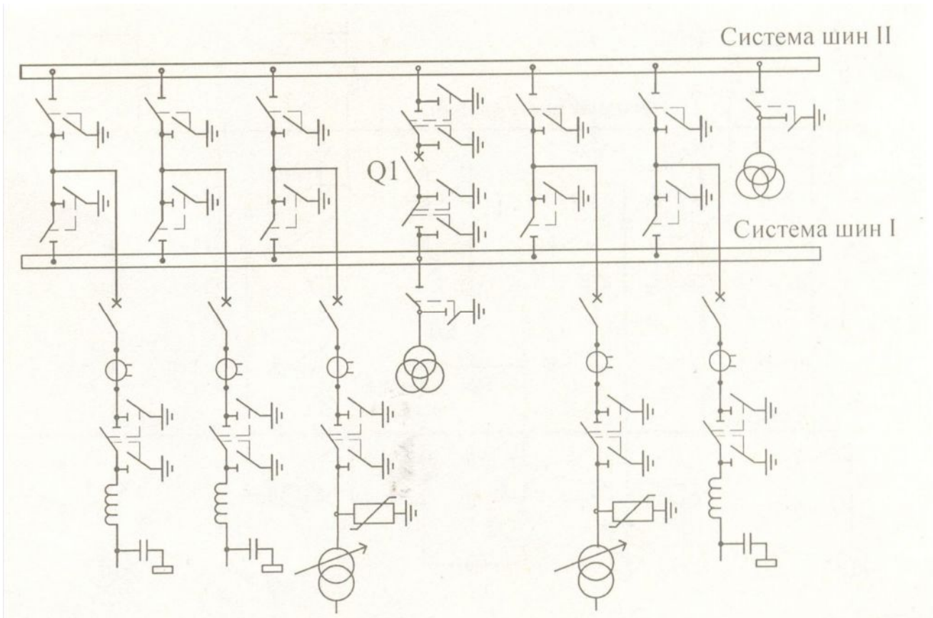
Схема с двумя системами шин с шиносоединительным выключателем Q1
