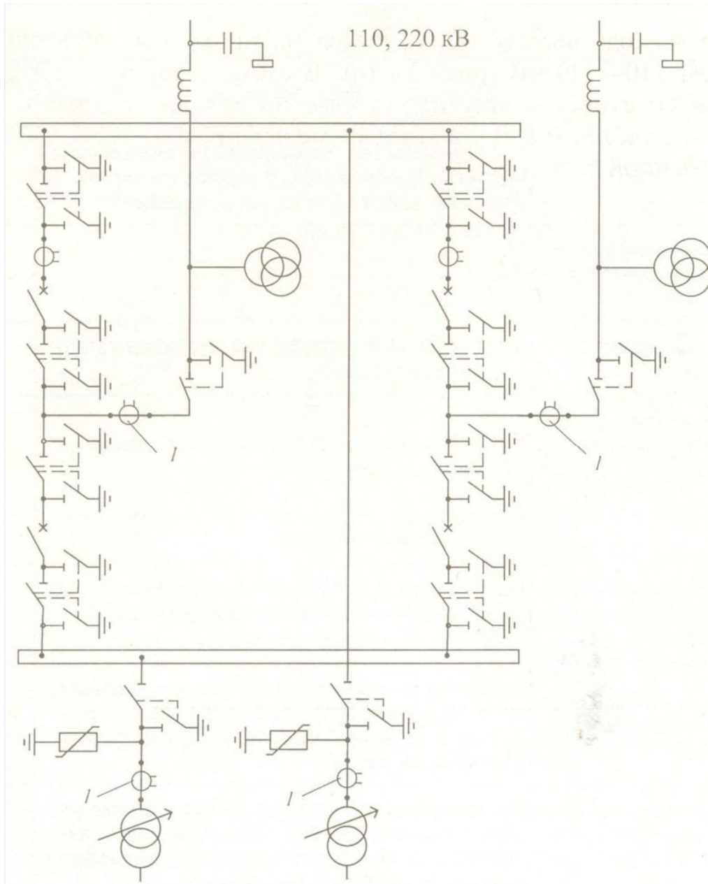
Схема четырехугольника: 1 - трансформаторы тока, установка которых должны быть обоснована (индекс схемы - 7 по [26])
