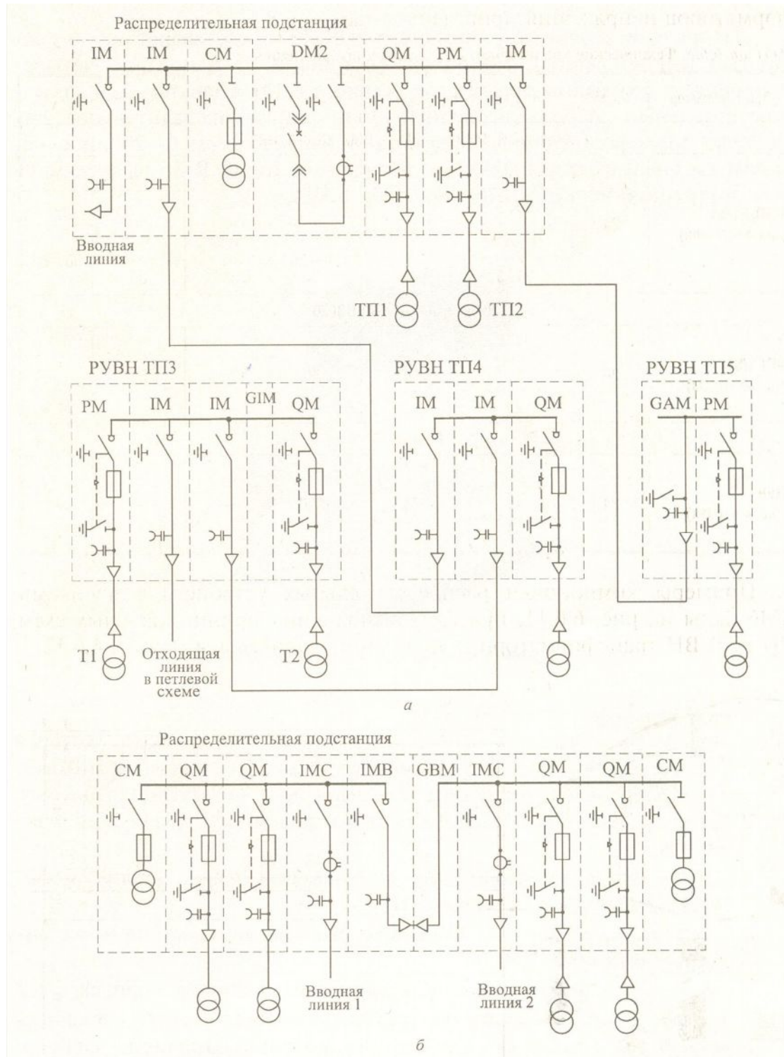
Примеры принципиальных схем РП и РУВН трансформаторных подстанций: а - распределительной сети; б - распределительной подстанции
