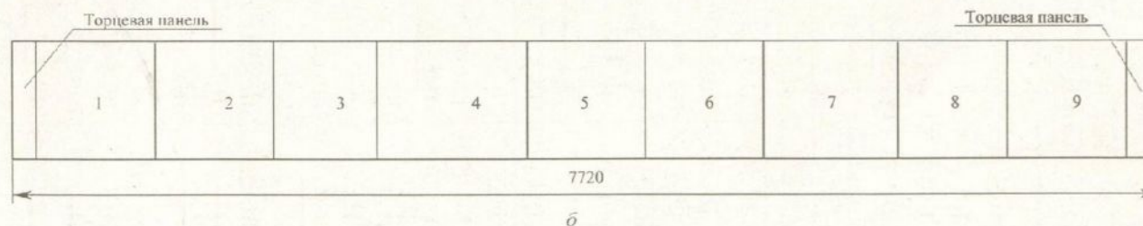
Схема (а) и план (б) распределительного устройства напряжением 380/220 Вольт с панелями ЩО-70-1
