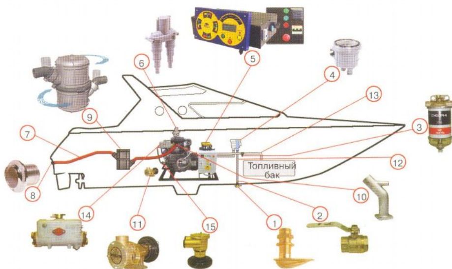
Типовая схема установки с дополнительным оборудованием
