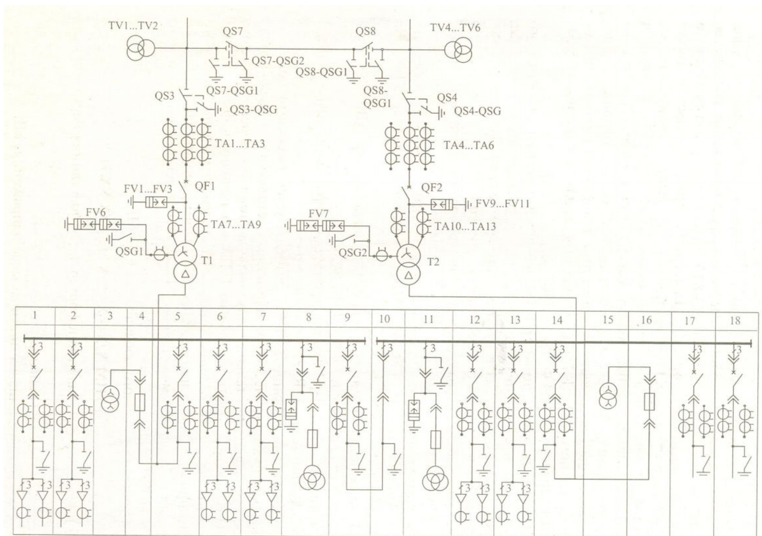
Схема электрическая принципиальная главных цепей КТПБ-10000, 16000/110/6(10) У1
