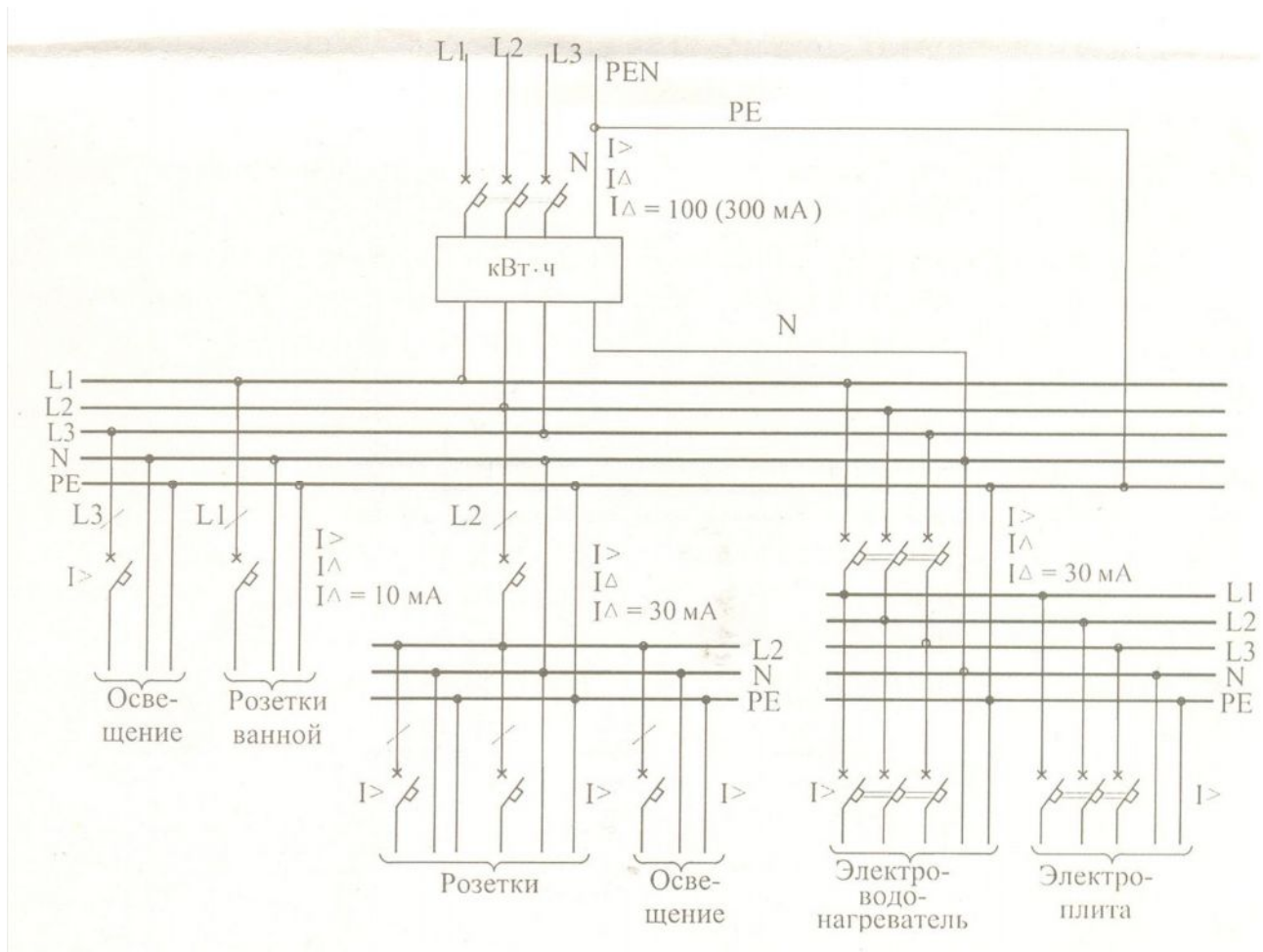
Схема электроснабжения квартиры повышенной комфортности с трехфазным вводом с системой TN-C-S
