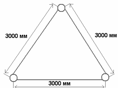
Контур заземления (вид сверху)
