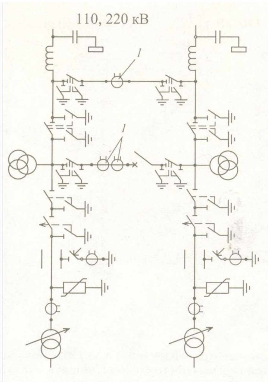
Схема «мостик с выключателем в перемычке и отделителями в цепях трансформаторов»: 1 - трансформаторы тока, установка которых должны быть обоснована (индекс схемы - 5 по [26]) (Имеет ограниченное применение в сетях напряжением 110 кВ)
