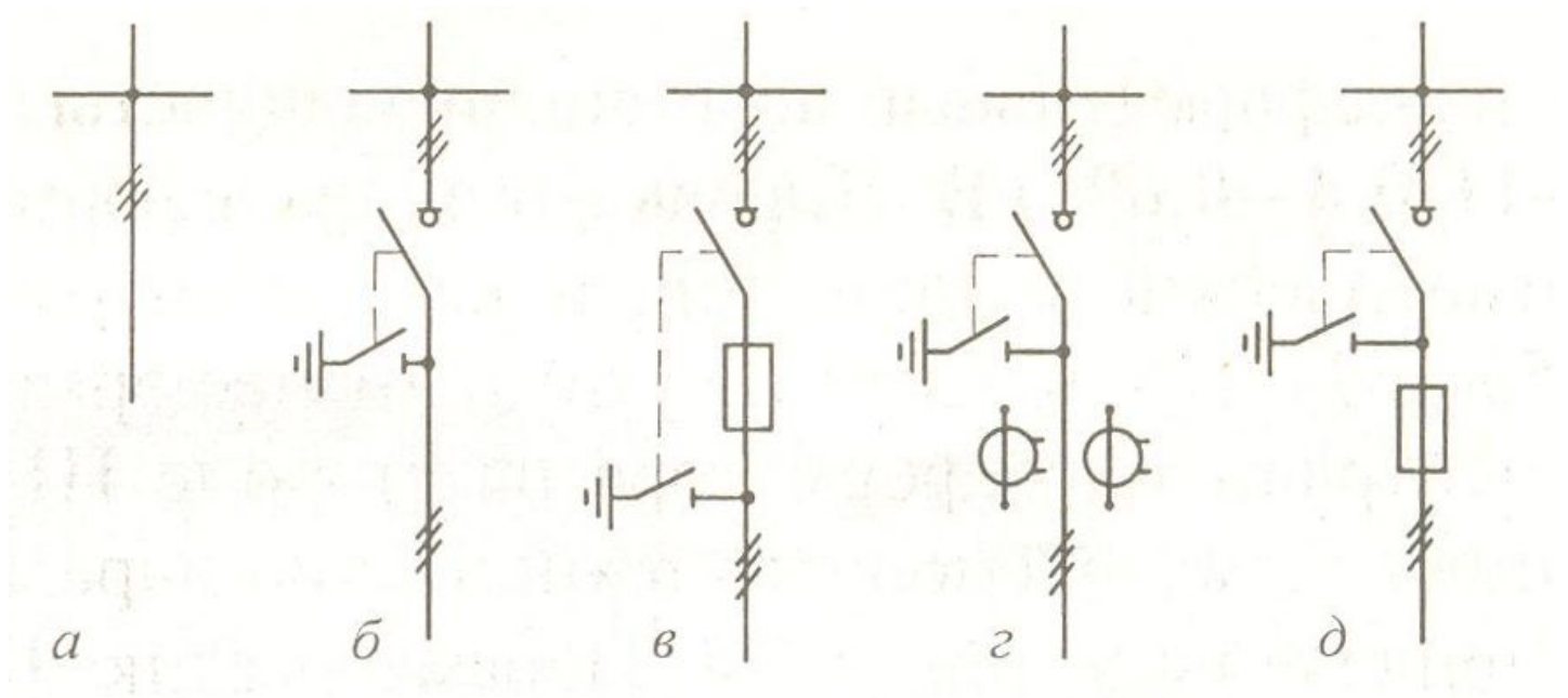
Однолинейные схемы главных цепей УВН КТП 630 и КТП 1000 Чирчикского трансформаторного завода: а - ВВ-1; б - ШВВ-2 -; в - ШВВ-2-2; г - ШВВ-2-3; д - ШВВ-3
