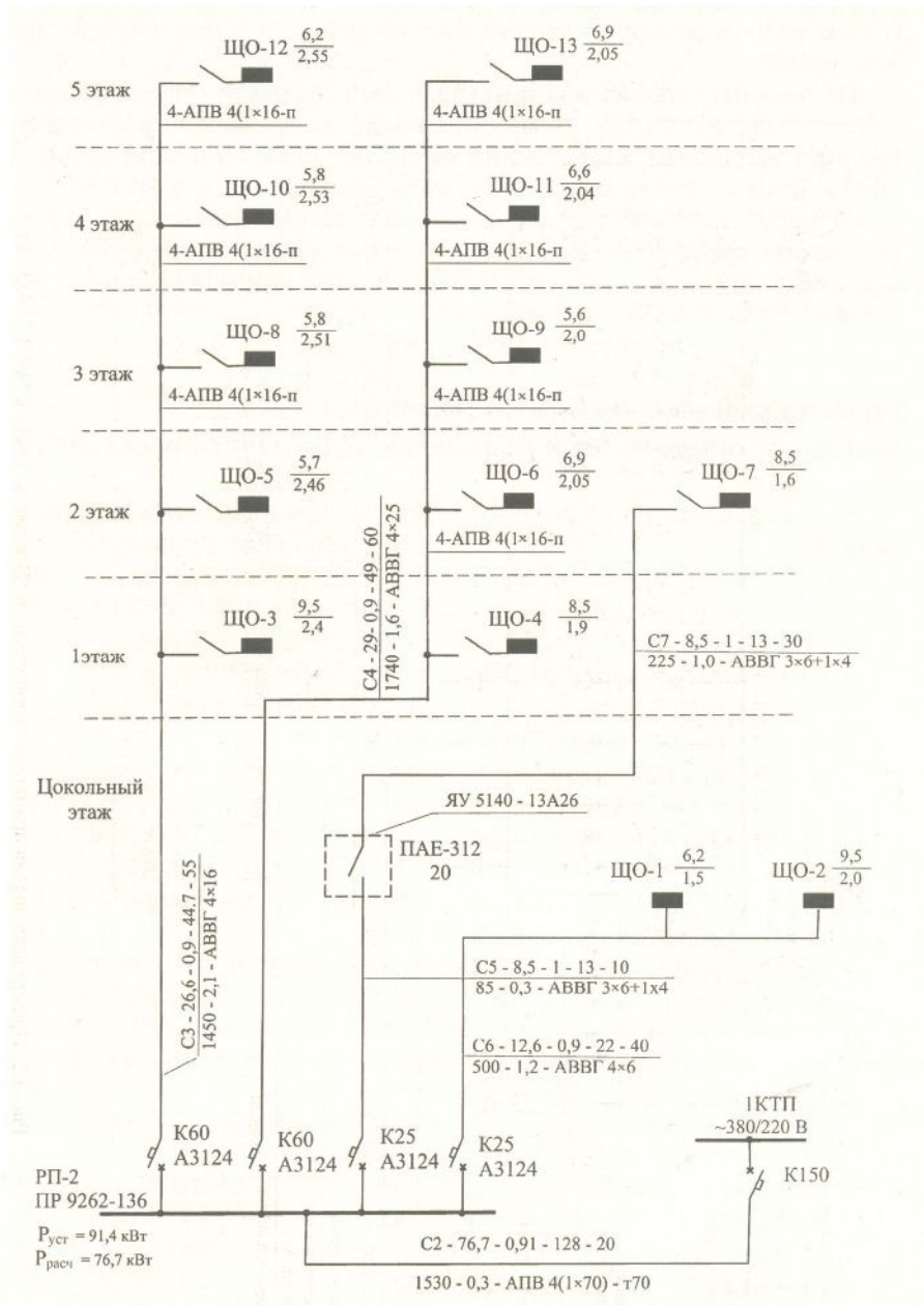
Пример оформления принципиальной схемы питающей сети многоэтажного здания по ГОСТ 21.608-84
