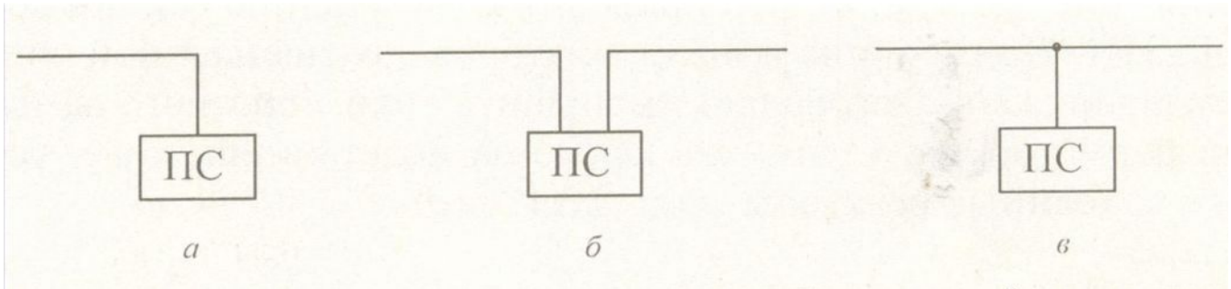
Схемы присоединения подстанций к питающей линии: а - тупиковая; б - проходная; в - ответвительная
