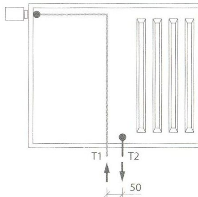
Левосторонне подключение
