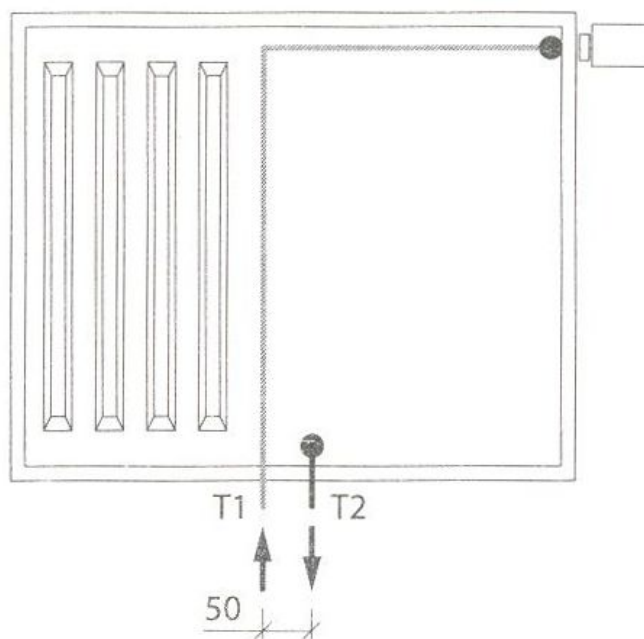
Стандартное подключение
