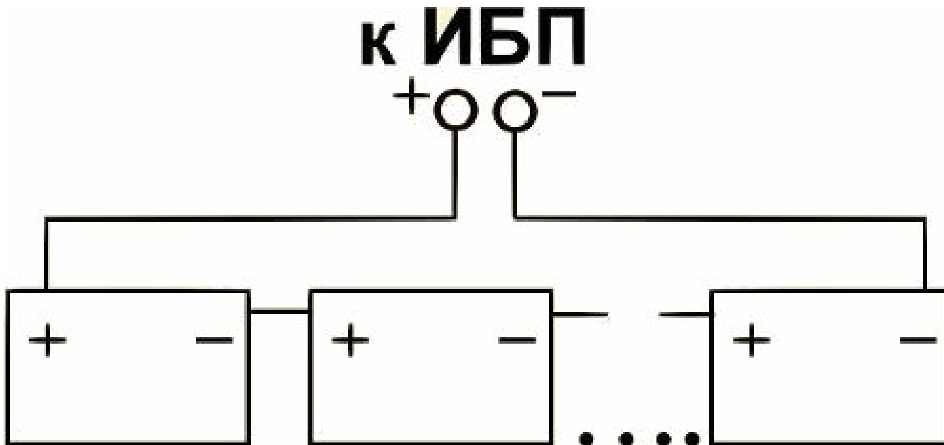
Схема последовательного подключения аккумуляторов к ИБП
