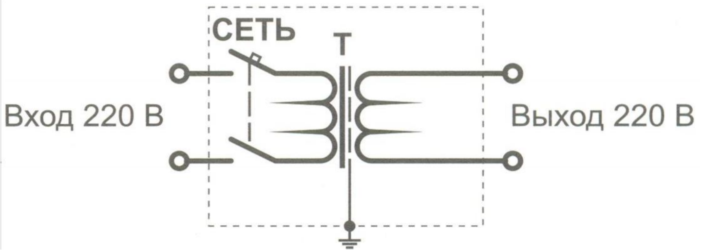
Трансформатор разделительный (принципиальная схема)
