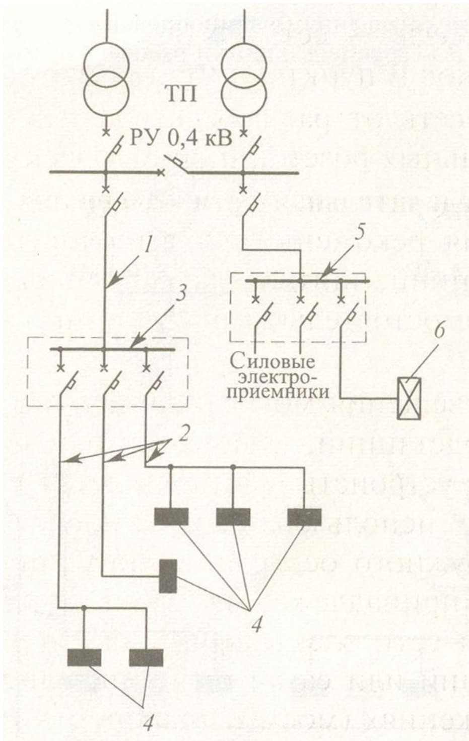
Схема питающей и распределительной сети освещения: 1 - питающая сеть; 2 - распределительная сеть; 3 - щит рабочего освещения; 4 - групповые щитки рабочего освещения; 5 - распределительный пункт; 6 - щиток аварийного освещения
