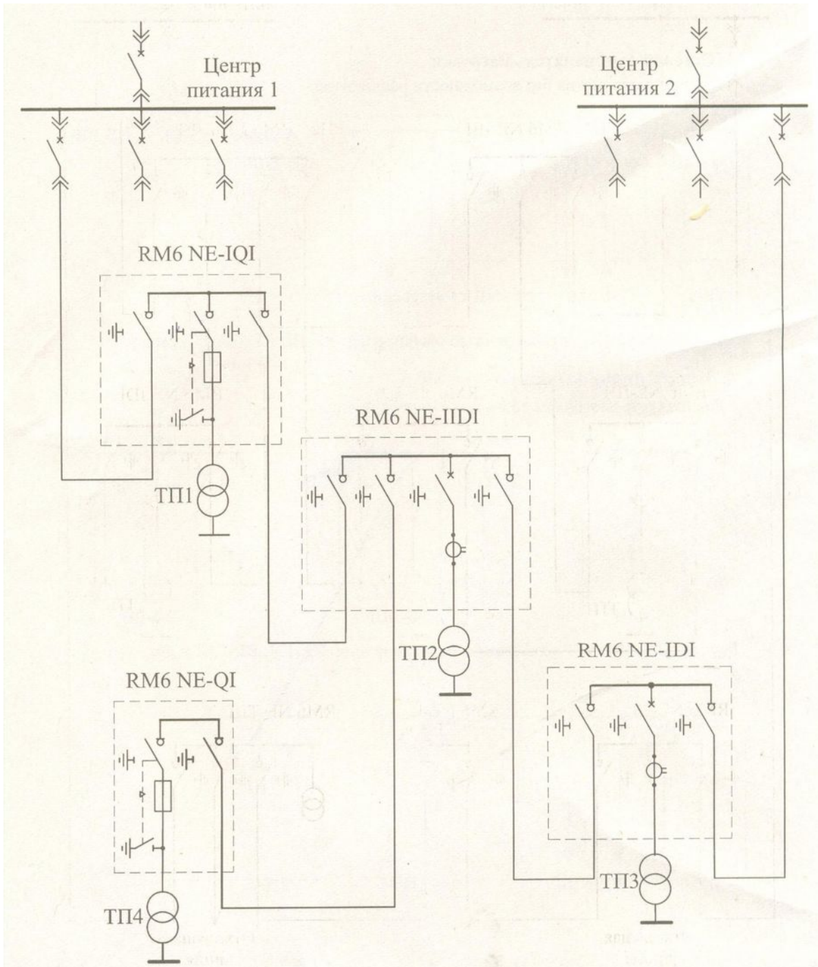
Пример выполнения петлевой схемы распределительной сети с моноблоками RM6
