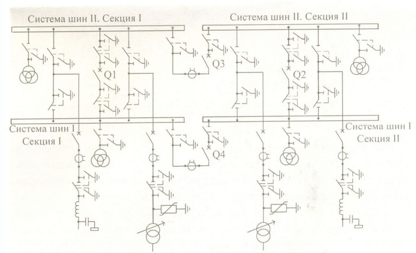
Схема с двумя секционированными системами шин с двумя шиносоединительными (Q1, Q2) и двумя секционными (Q3, Q4) выключателями
