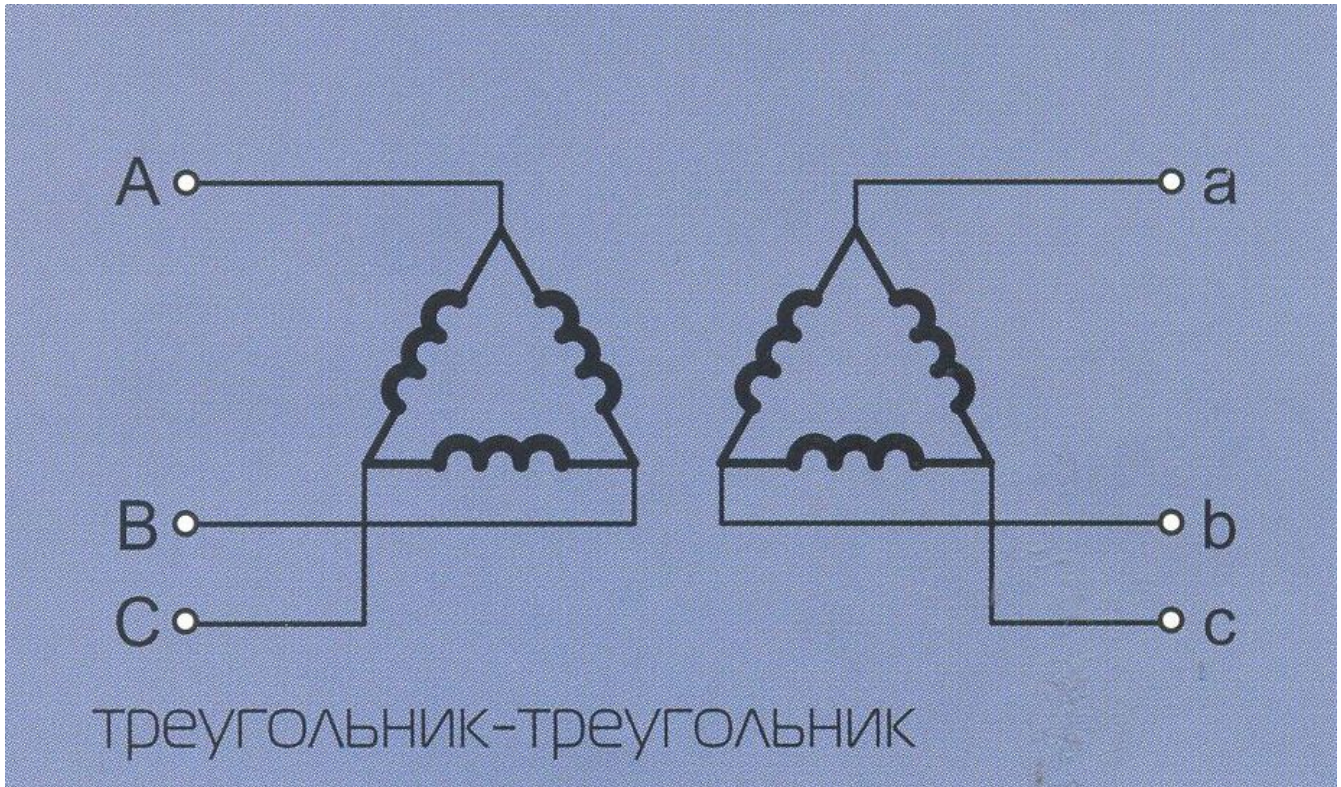
Схема подключения трехфазных потребителей типа «треугольник-треугольник»
