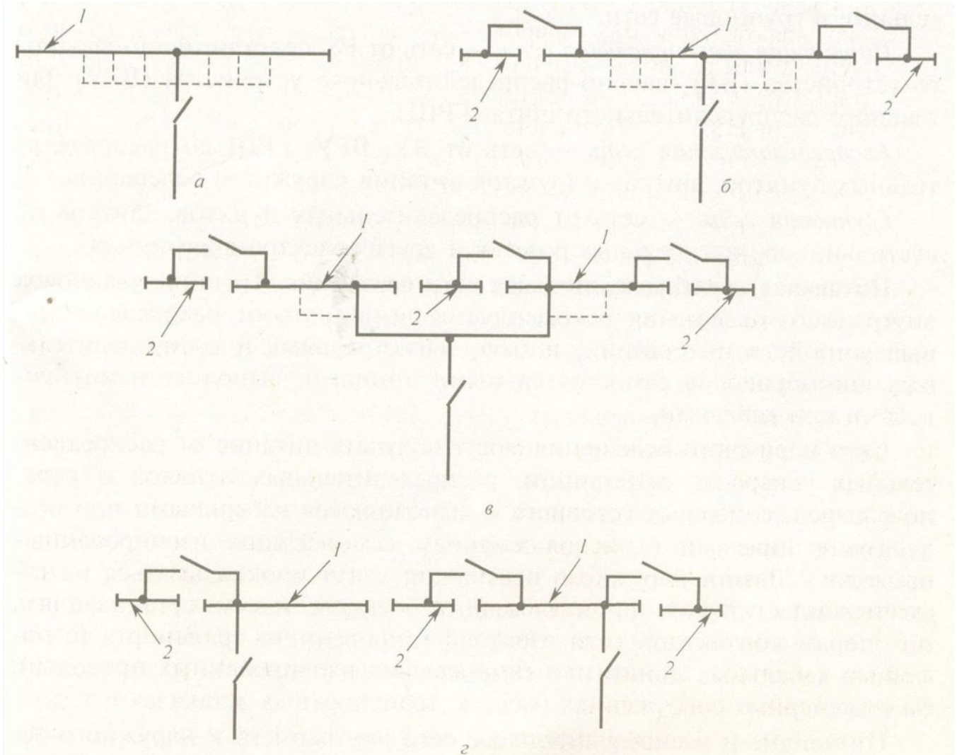
Схемы троллейных линий: а - несекционированная; б - с двумя ремонтными секциями; в, г - с тремя ремонтными секциями; 1 - троллейная линия; 2 - ремонтные секции
