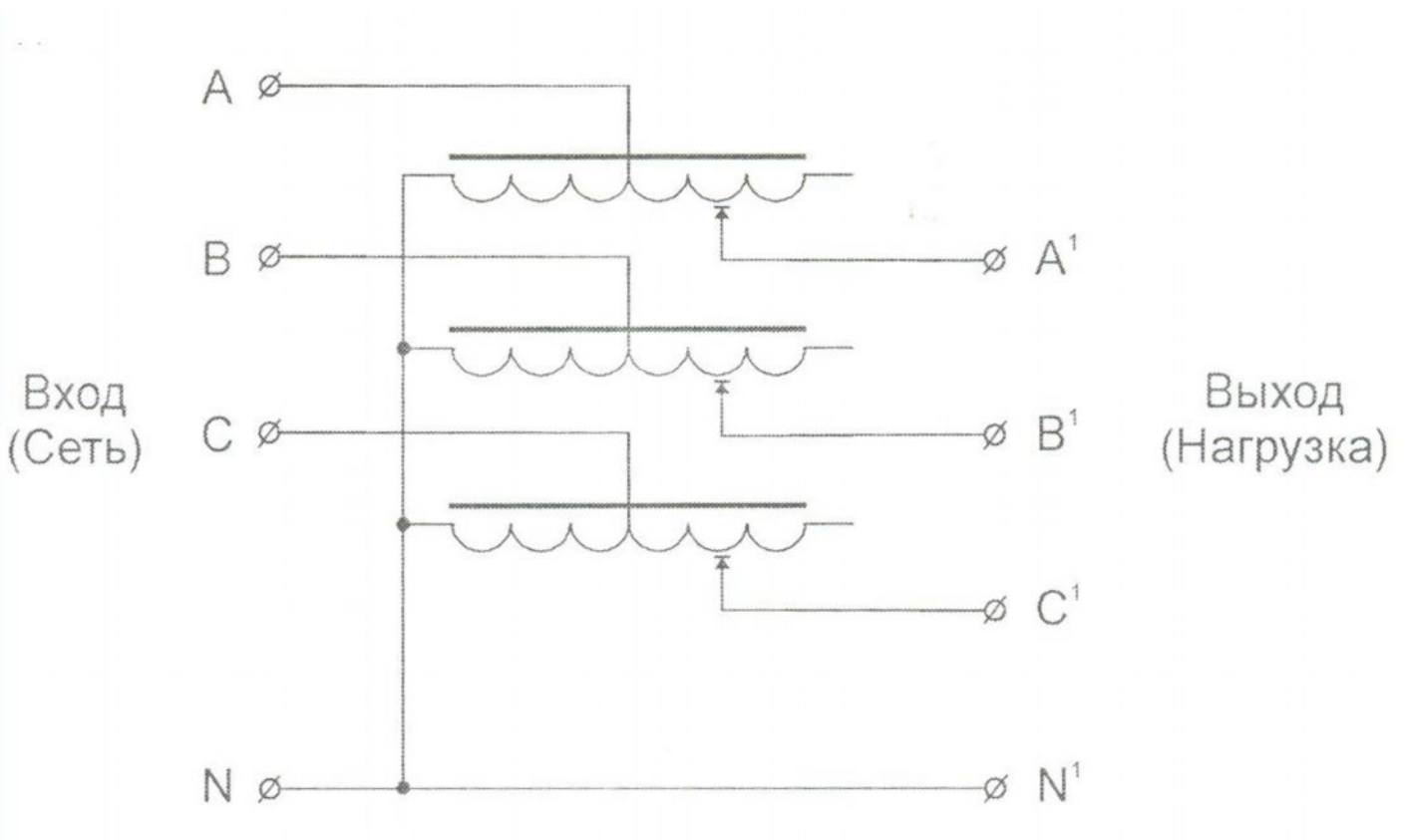
Схема включения автотрансформатора
