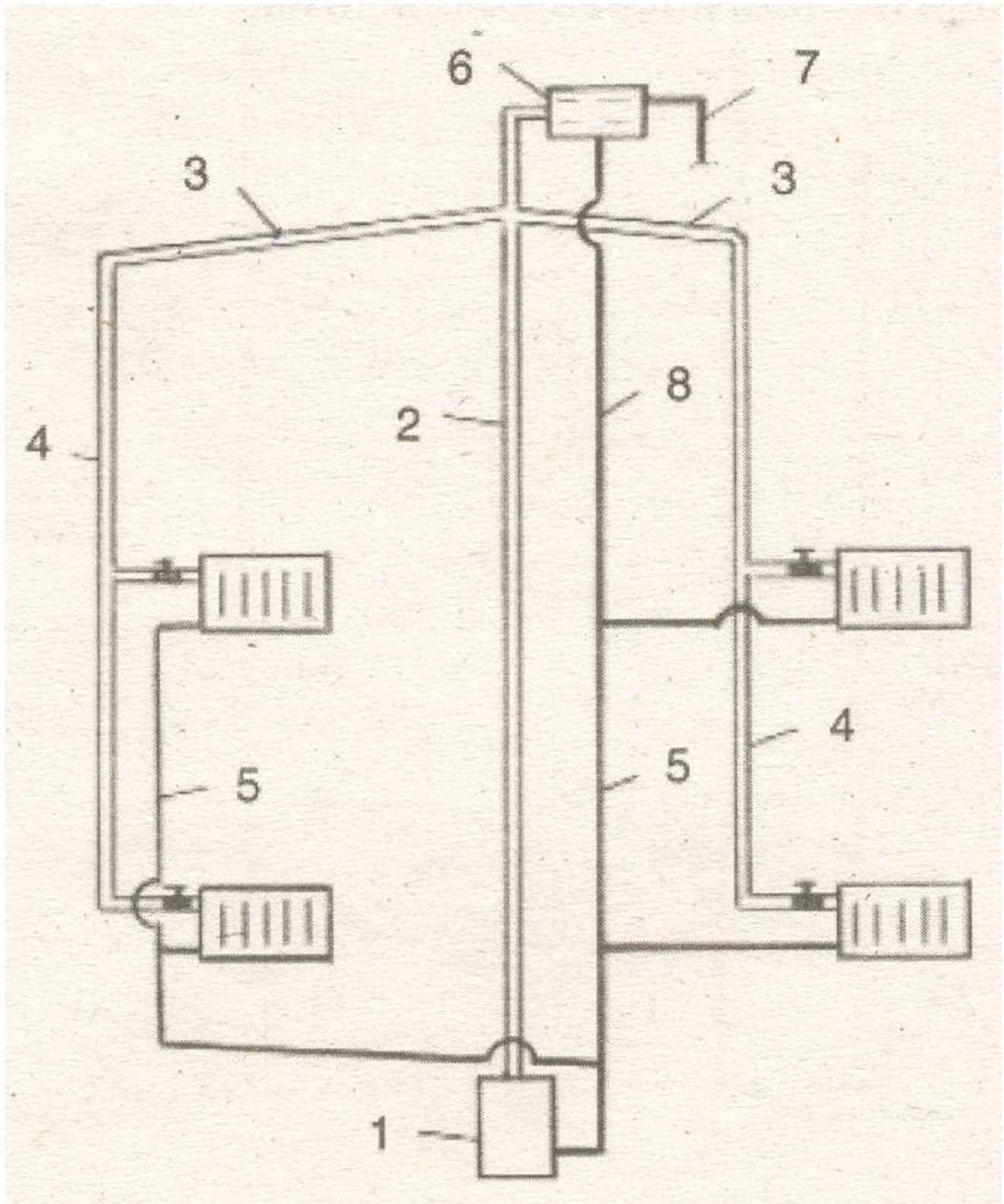
Двухтрубная система водяного отопления с принудительной циркуляцией. Фрагмент с верхней разводкой: 1 - отопительный котел ; 2 - главный стояк; 3 - разводящие трубопроводы горячей воды; 4 - стояки горячей воды; 5 - обратные стояки; 6 - расширительный бак ; 7 - переливная труба; 8 - предохранительный трубопровод.
