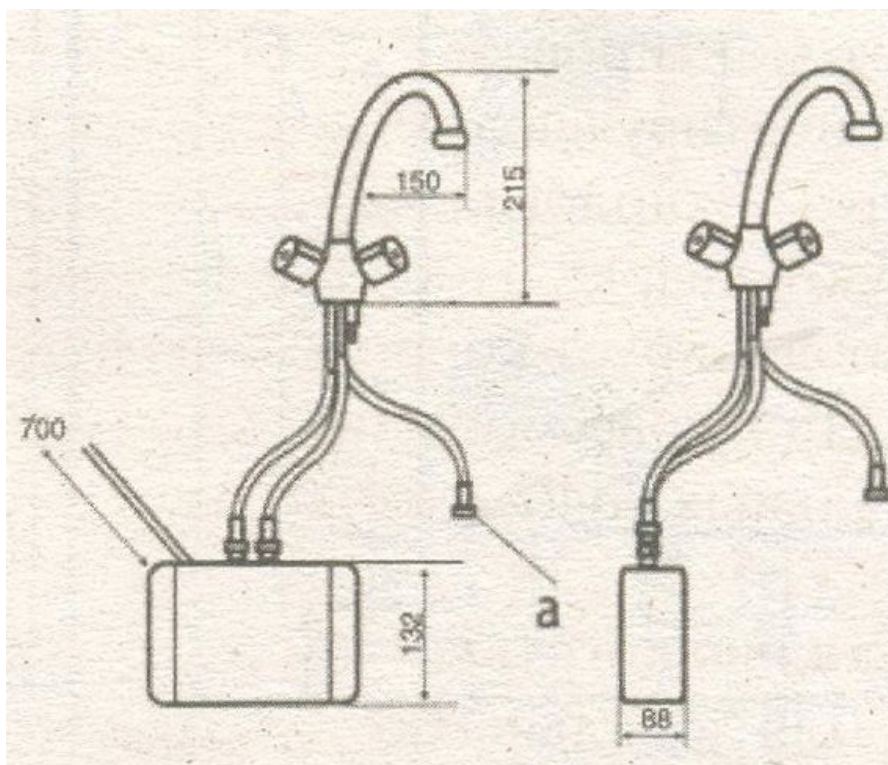
Схемы водонагревателей UDM...U (а - вход холодной воды)
