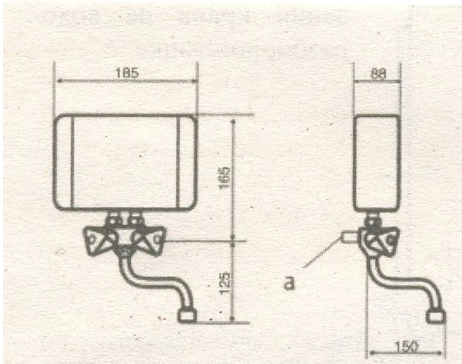
Схемы водонагревателей UDM (а - вход холодной воды)
