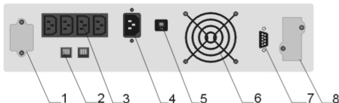
а) ДПК-1/1-1-220-Т
