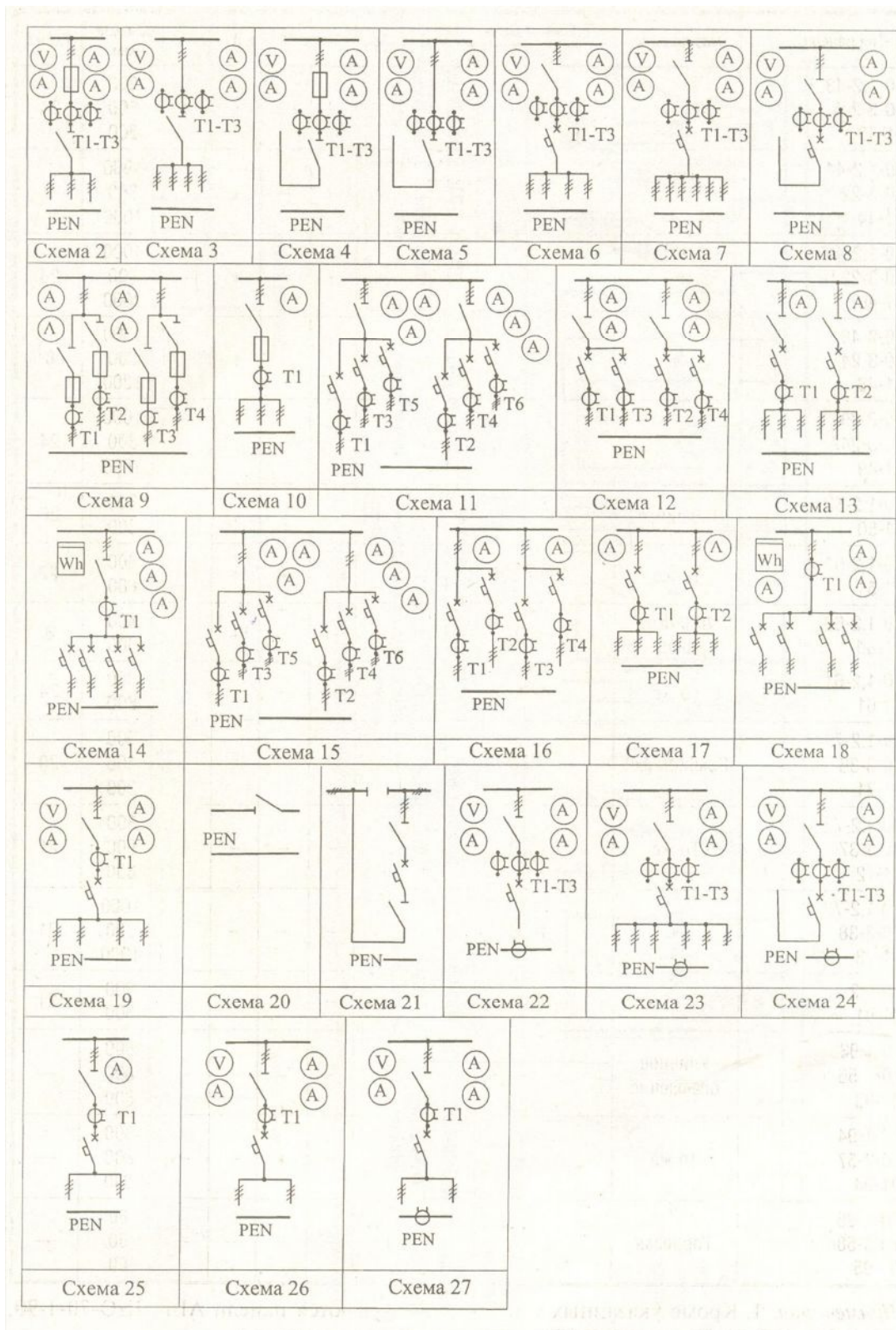
Схемы первичных соединений панелей ЩО-70-1; ЩО-70-2; ЩО-70-3, ЩО-01 производства ЗАО ПК «ИЗНУ»
