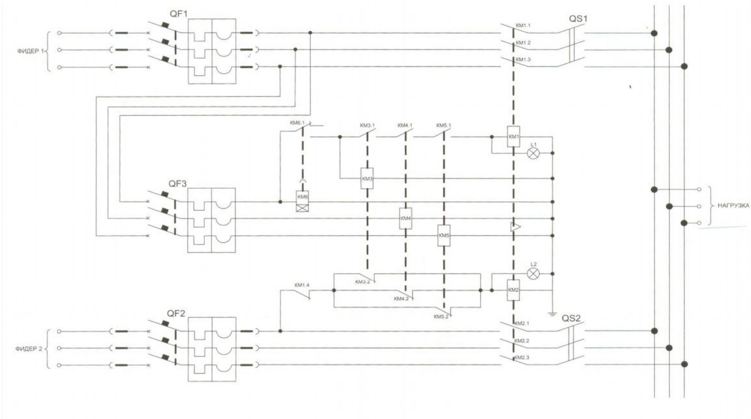
Структурная схема ШАВР-0,4 исполнения РЛ
