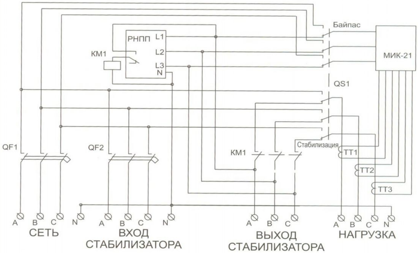
Структурная схема трехфазного щита ЩК-0,4-3
