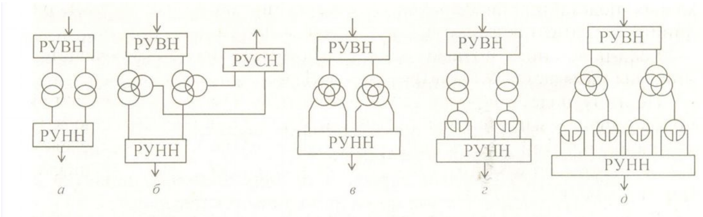
Структурные схемы трансформаторных подстанций
