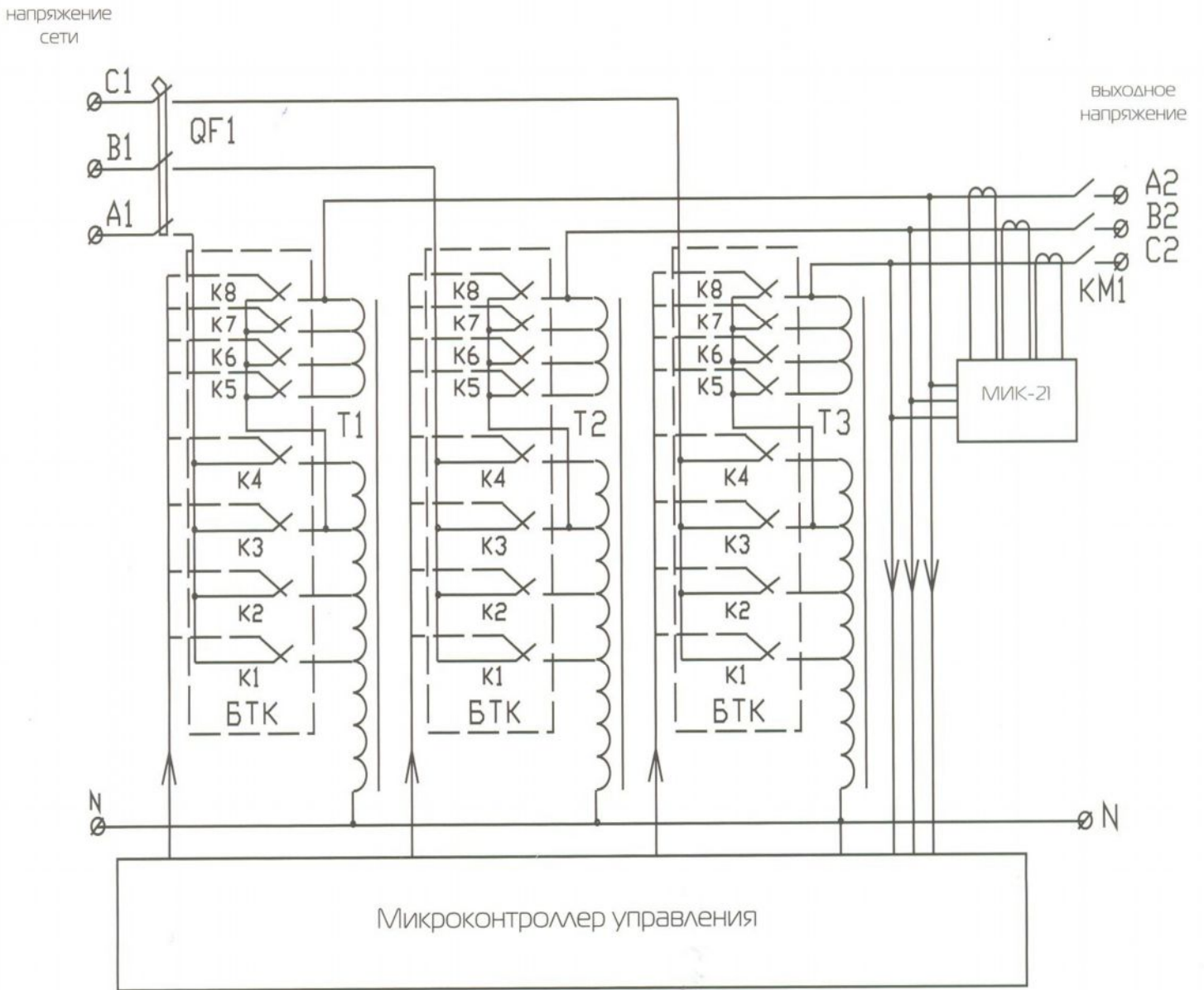
Структурная схема трехфазного стабилизатора напряжения СДТ
